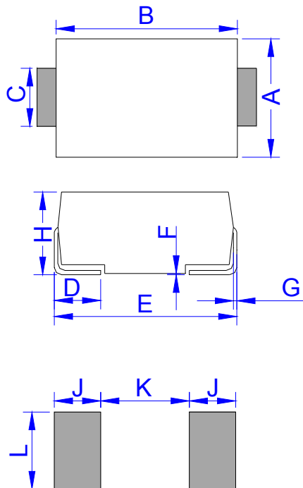
DO-214AC (SMA)
